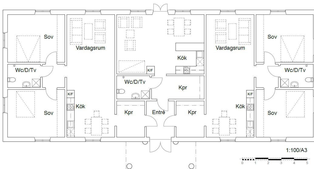
Flefamiljhus 1-plan skiss 20.03.10
