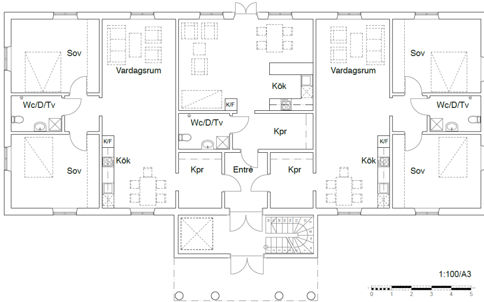
Flefamiljhus 2-plan skiss 20.03.10
